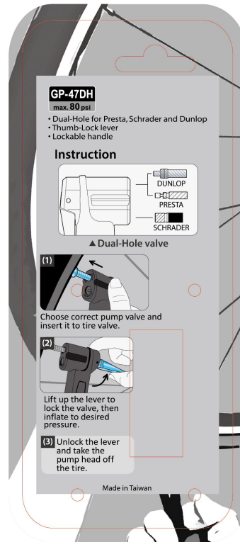
※刀模同(GP47L,GP47E) 113/04/25
